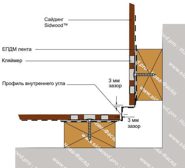
Профиль внутреннего угла
