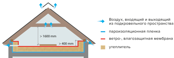
Рис. 1.8. Устройство вентиляции холодного чердака
