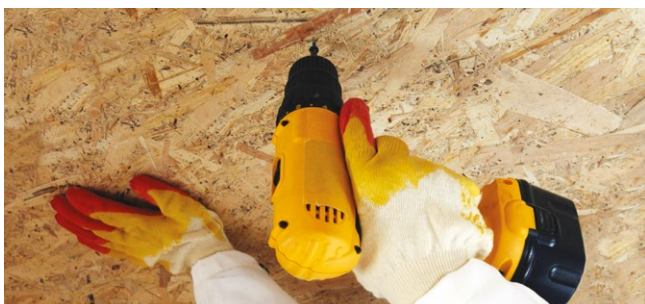
Рис. 1.10. Подшивка потолка листами ОСП
