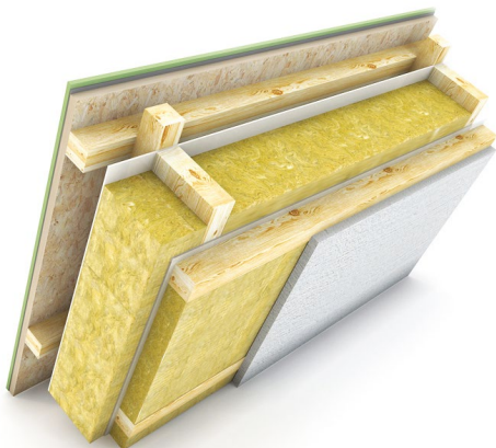
Рис. 1.7. Устройство мансарды
