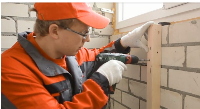
Рис. 3.1. Установка вертикального каркаса под теплоизоляцию
