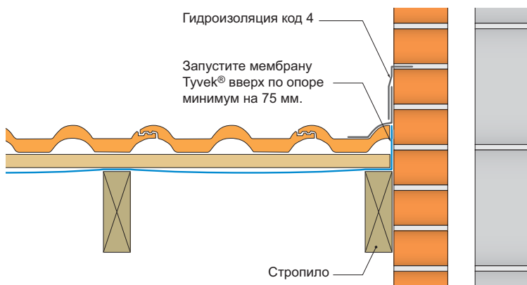
Рис. 43 - Опора
